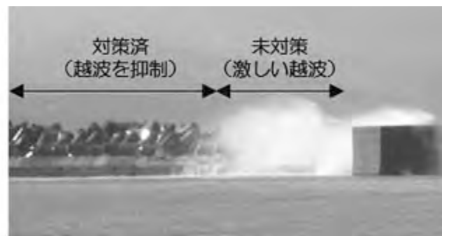
消波ブロック嵩上げによる越波抑制効果例
