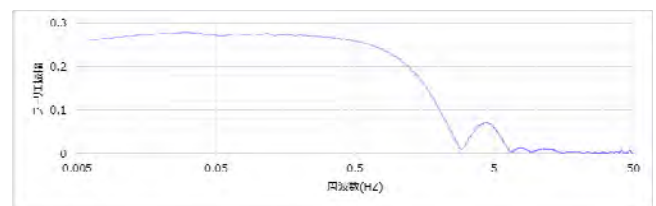
図-4 杭を変位させた際の振動特性
