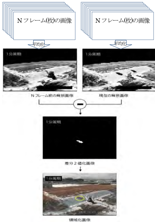
図-6 異常検知のイメージ
