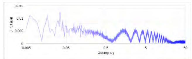
図-3 杭の付近を掘削した際の振動特性
